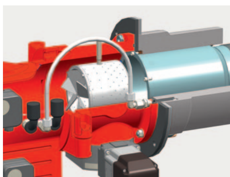
Specjalne przygotowanie mieszanki stwarza bezpieczne warunki podczas zapłonu
